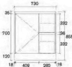
ASY-750W-SD Size: 730x455x855mm
